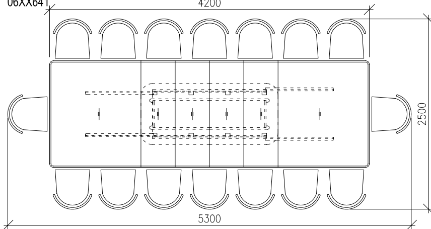
Stůl jídelní rozkládací - rozložený 4200 x 1400 x 760 mm 06XX641
